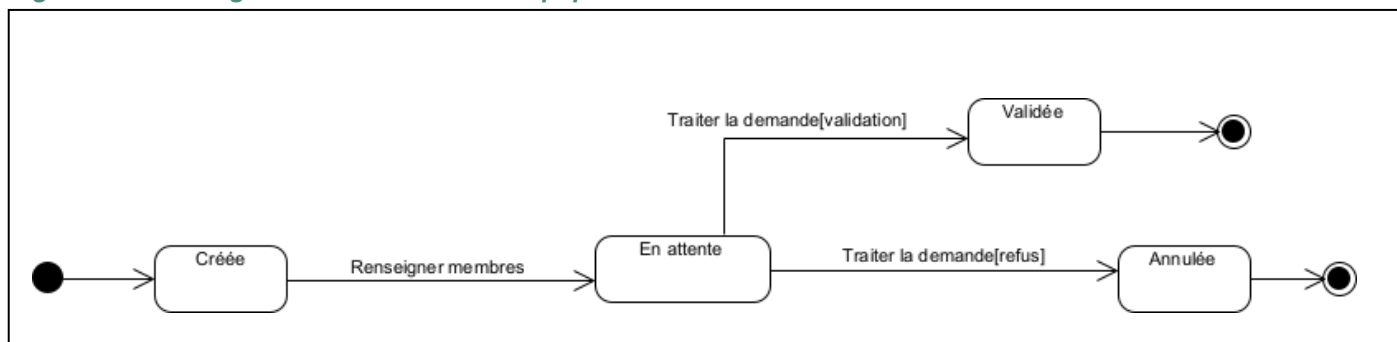
Figure 2.6 – Changements d'états d'une équipe
