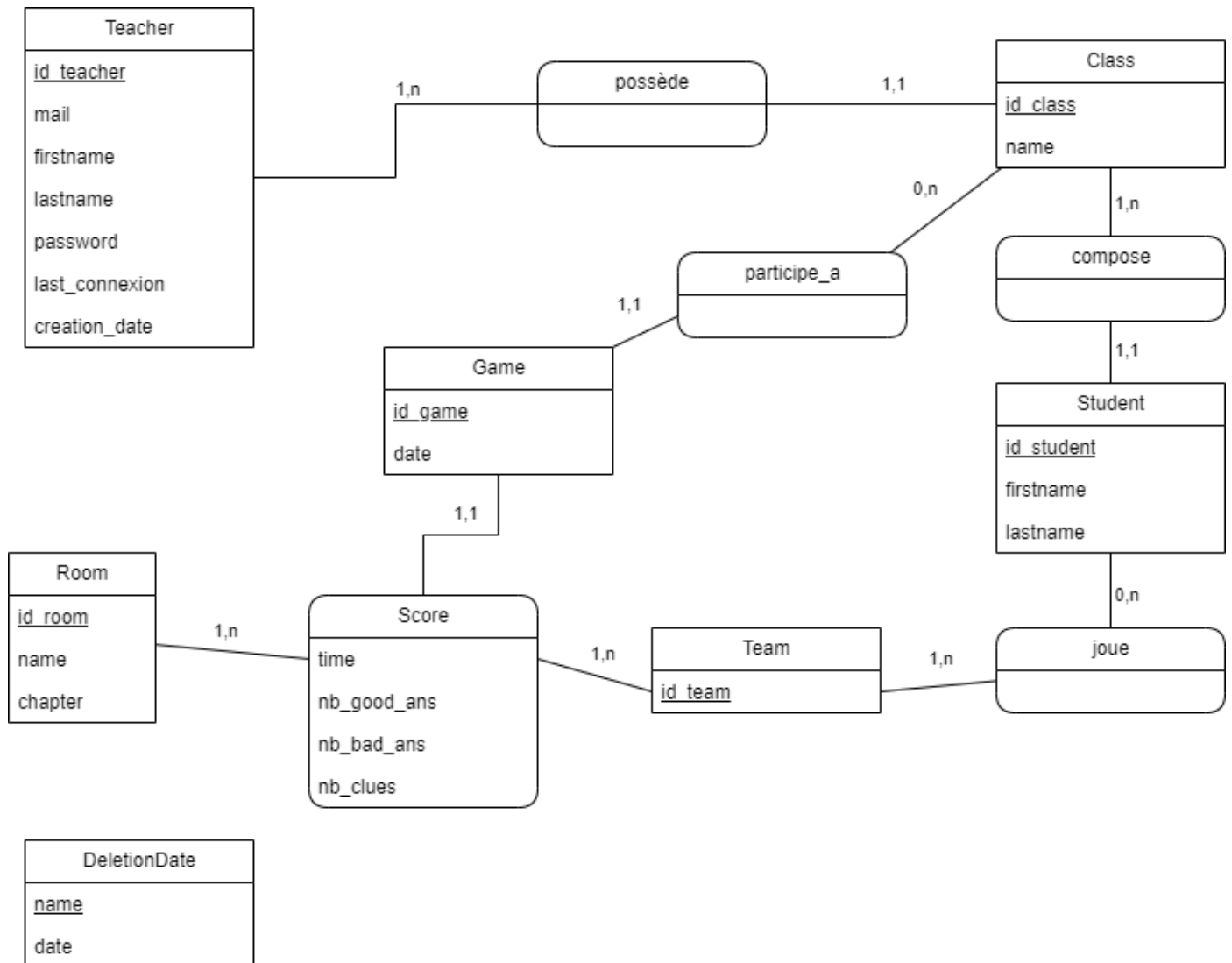
Figure 2.10 – Schéma Entité-Association
