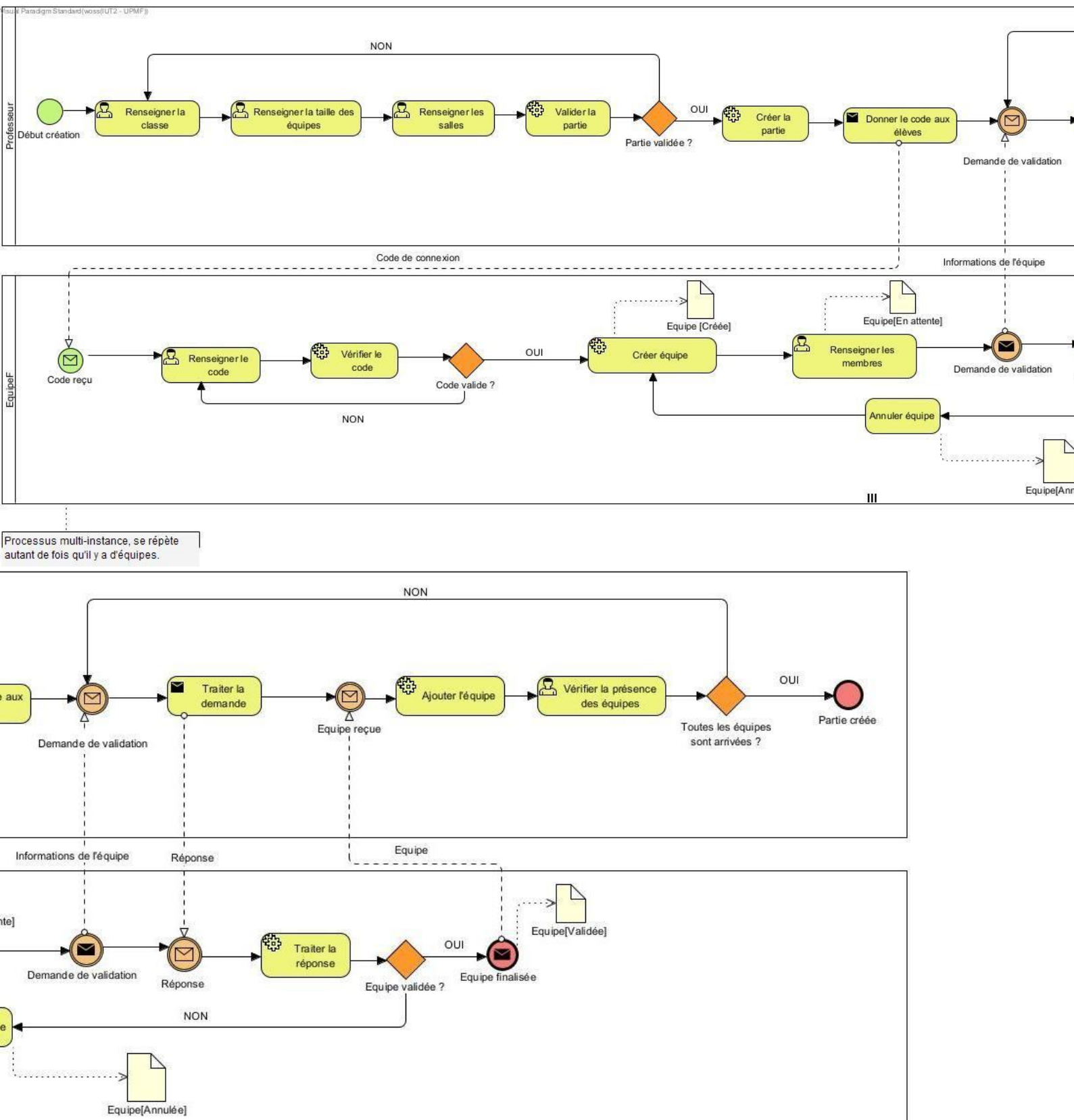
Figure 2.8 – Processus métiers – Créer une partie
