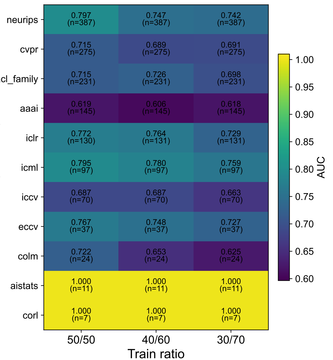
Arxiv ROC-AUC
