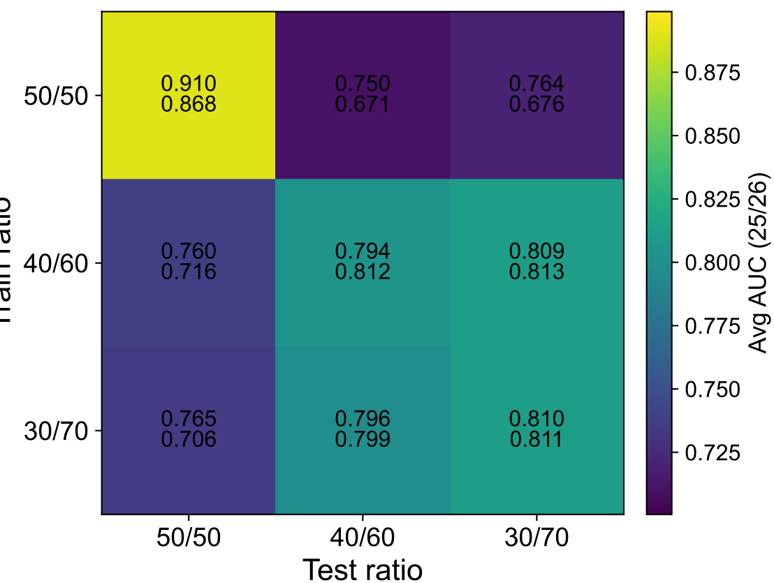
ICLR ROC-AUC
