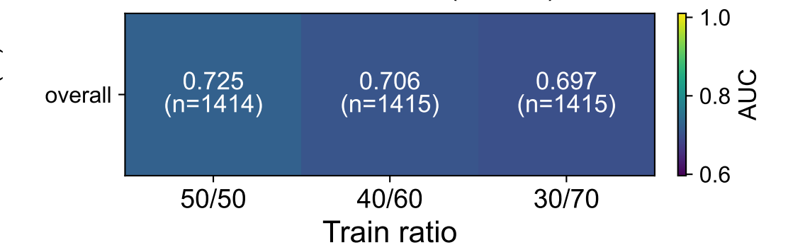
Arxiv ROC-AUC (overall)
