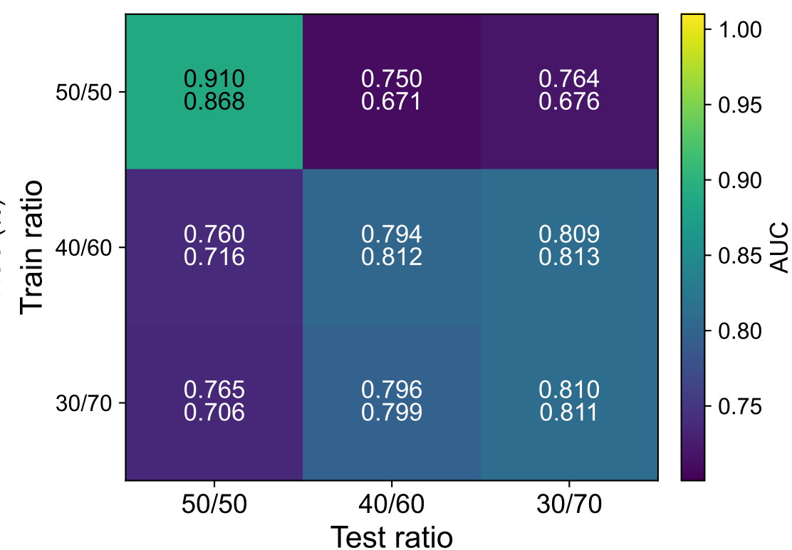
ICLR ROC-AUC
