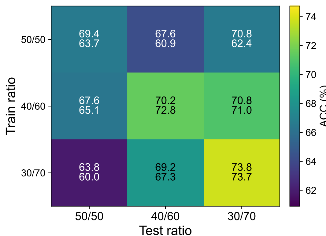
ICLR Raw ACC
