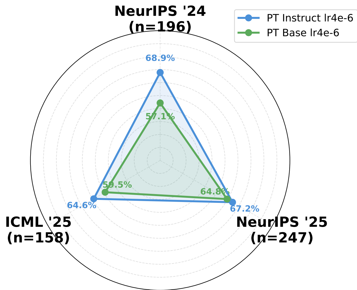
(d) Midtrain + SFT — Reject Recall
