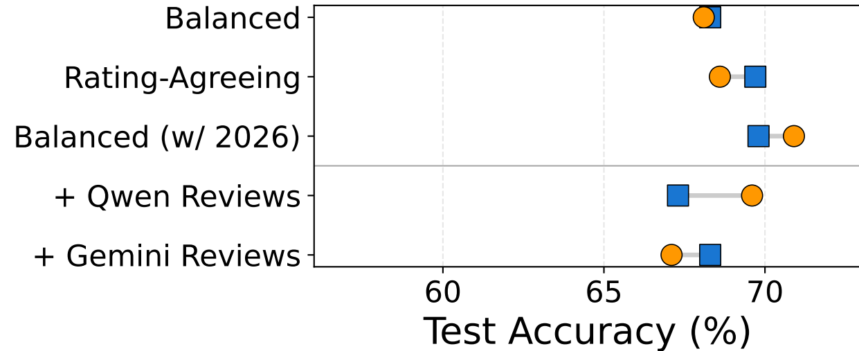
ICLR 2025
