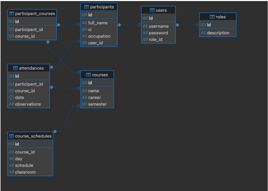
Figura 4.5: Diagrama de Entidad-Relación del sistema CheckFace[imagen propia].
