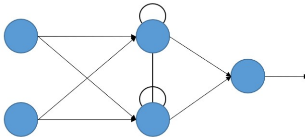
Figura 2.6: Representación de una red neuronal recurrente (RNN), donde las conexiones internas permiten el manejo de secuencias mediante memoria temporal [4].
