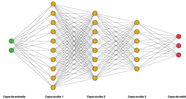
Figura 2.4: Estructura de una red neuronal profunda [3].
