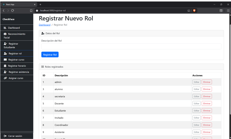
Figura 4.12: Gestión de roles: registro, edición y eliminación.
