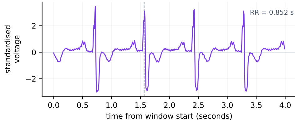
RBBB - MIT-BIH record 118
