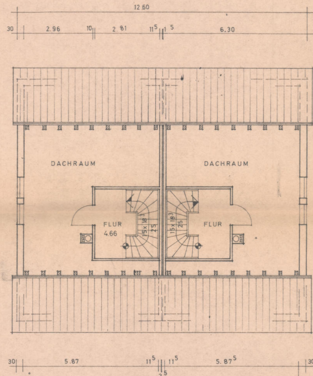
DACHGESCH
