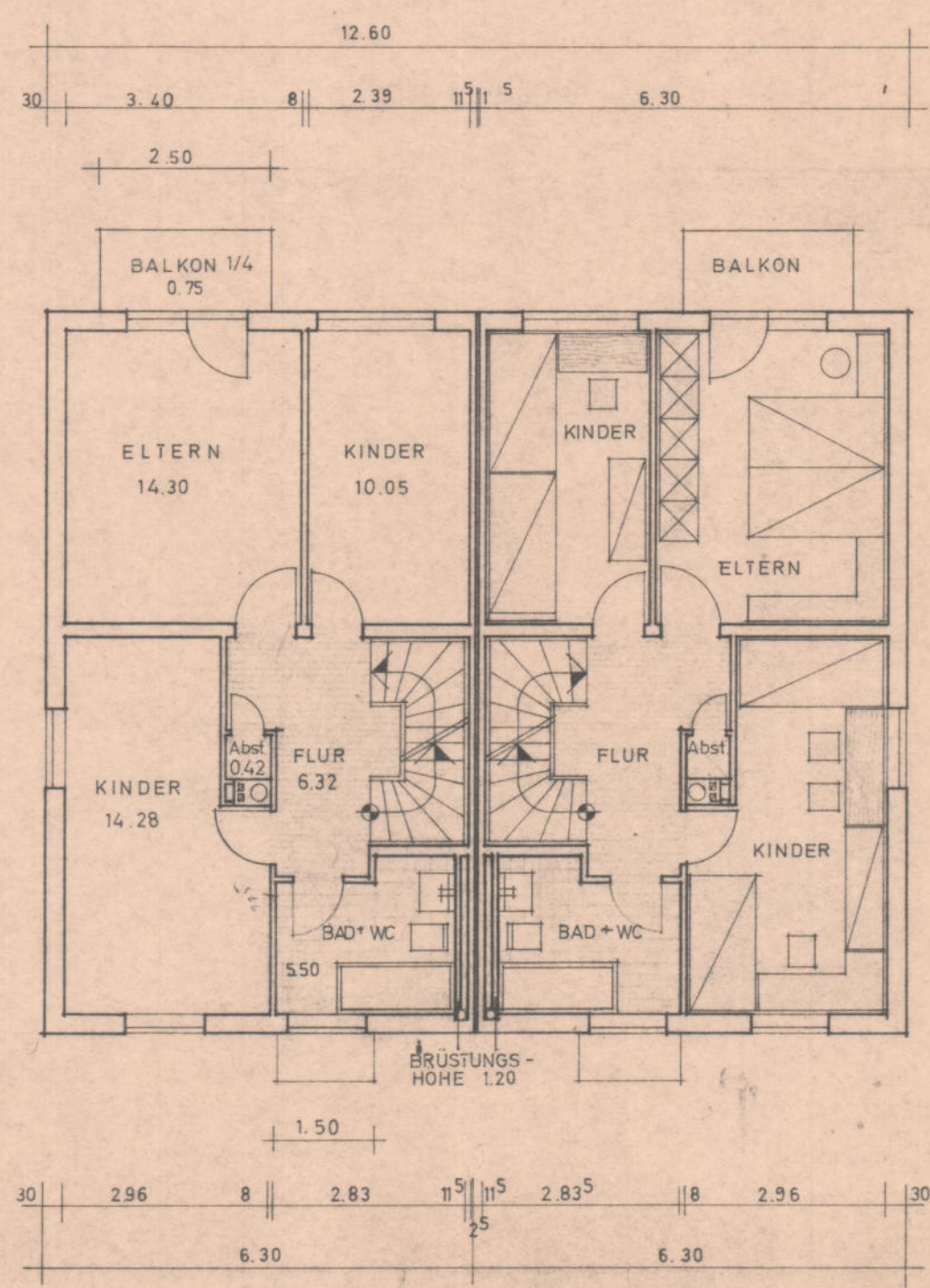
OBERGESCH
