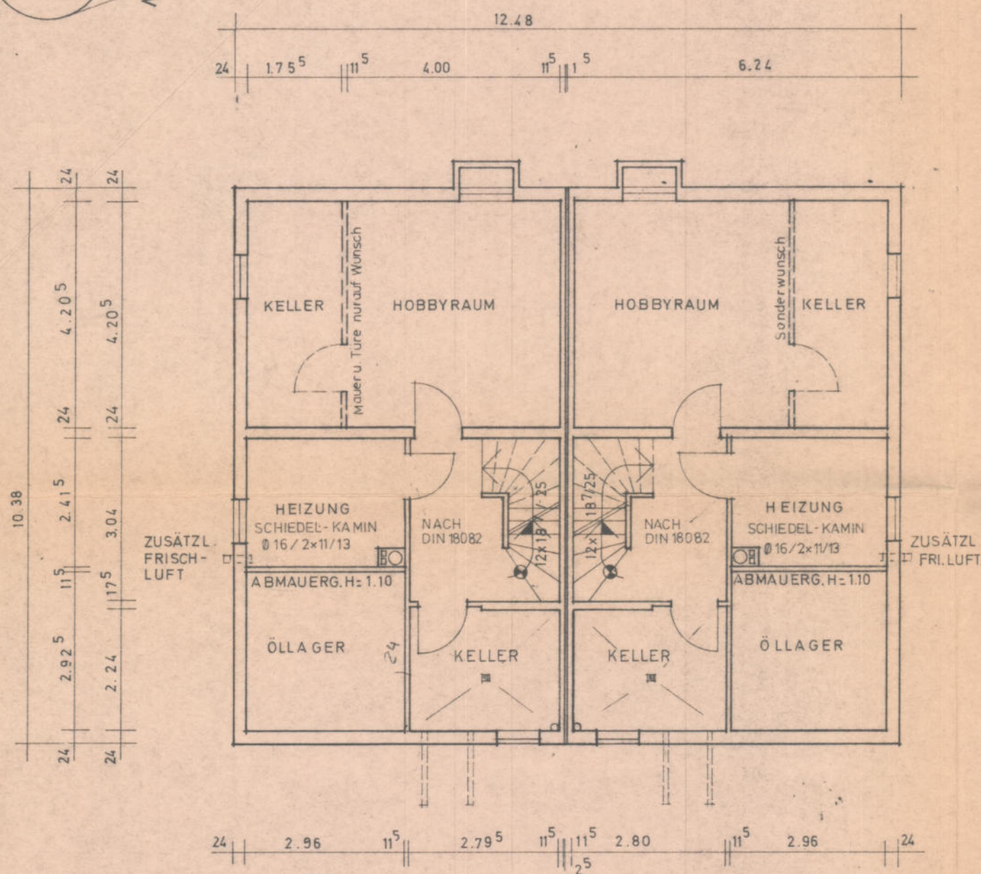
KELLERGESSCH
