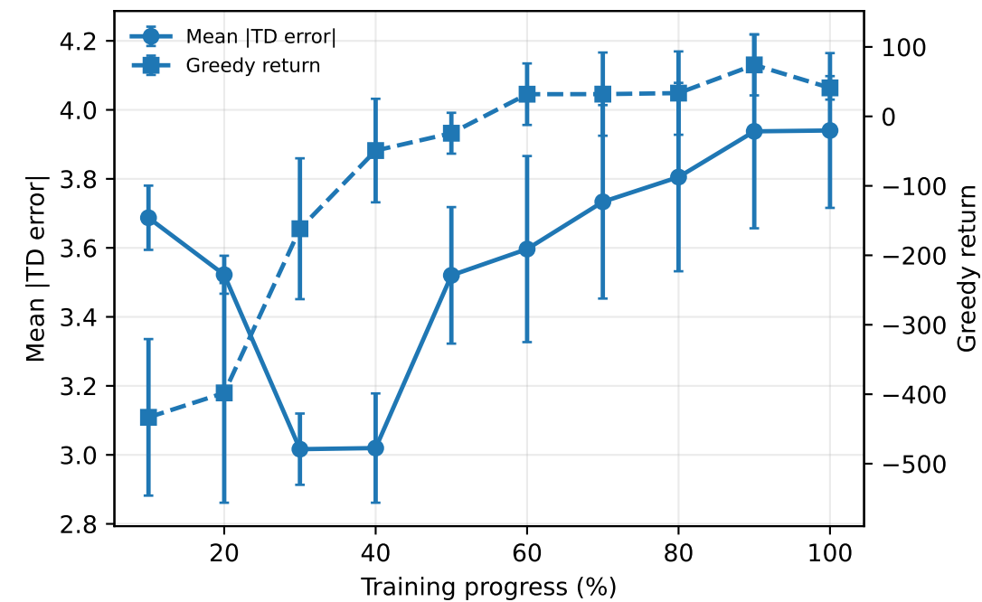
LunarLander
