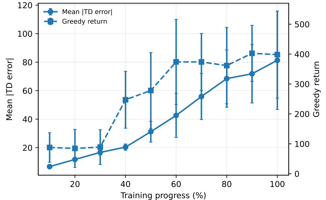
LunarLander
