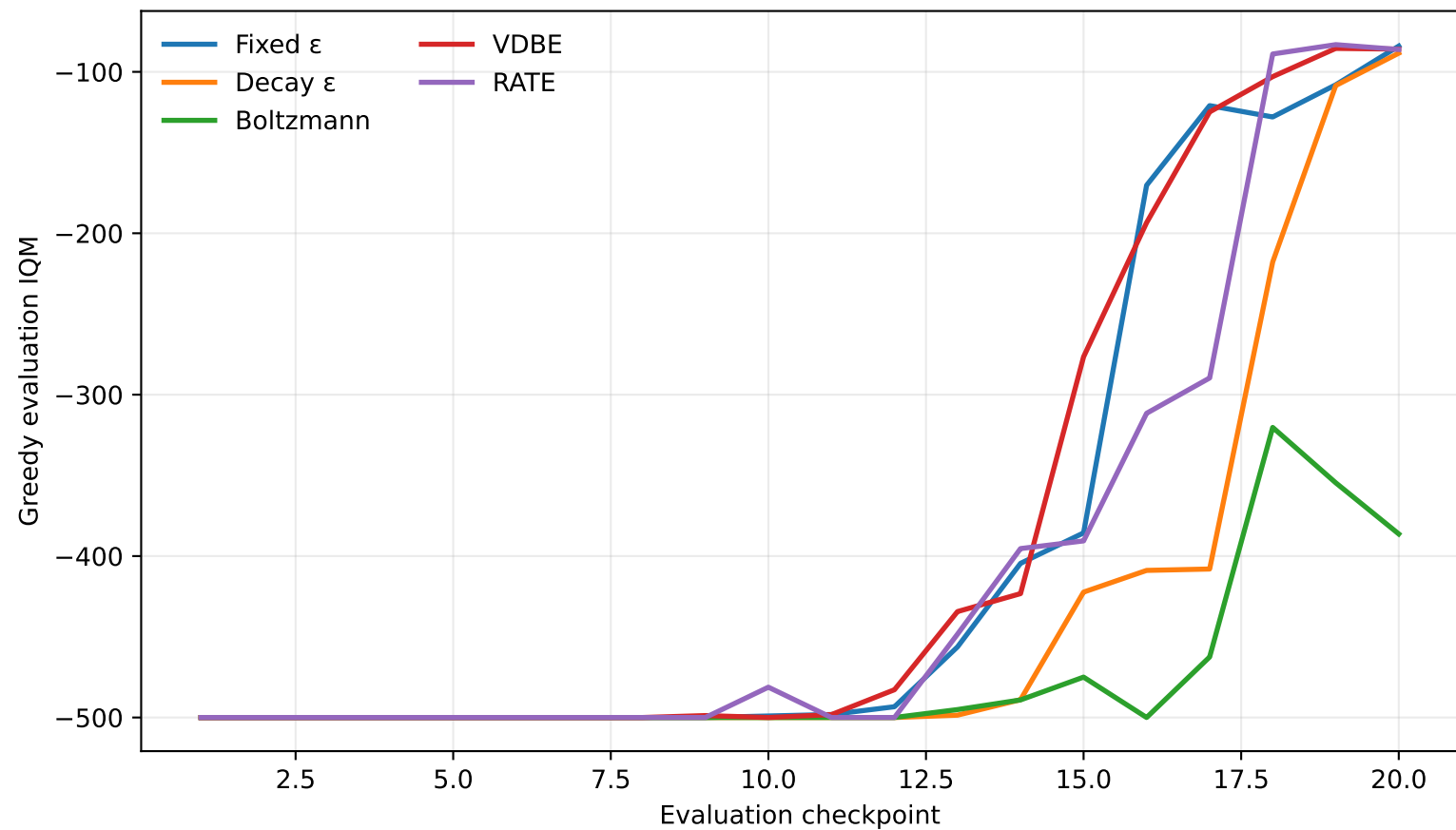
Acrobot — Double DQN
