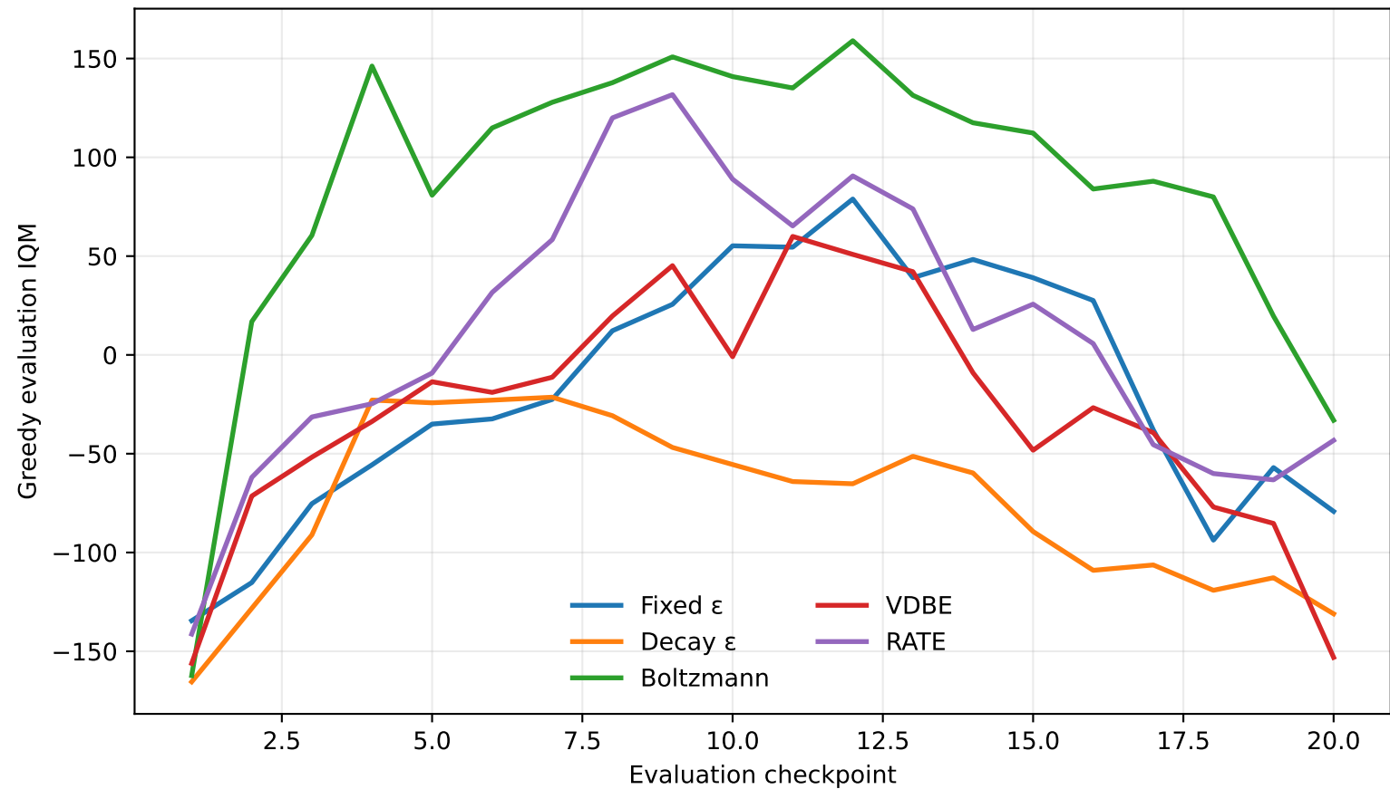
LunarLander — Double DQN
