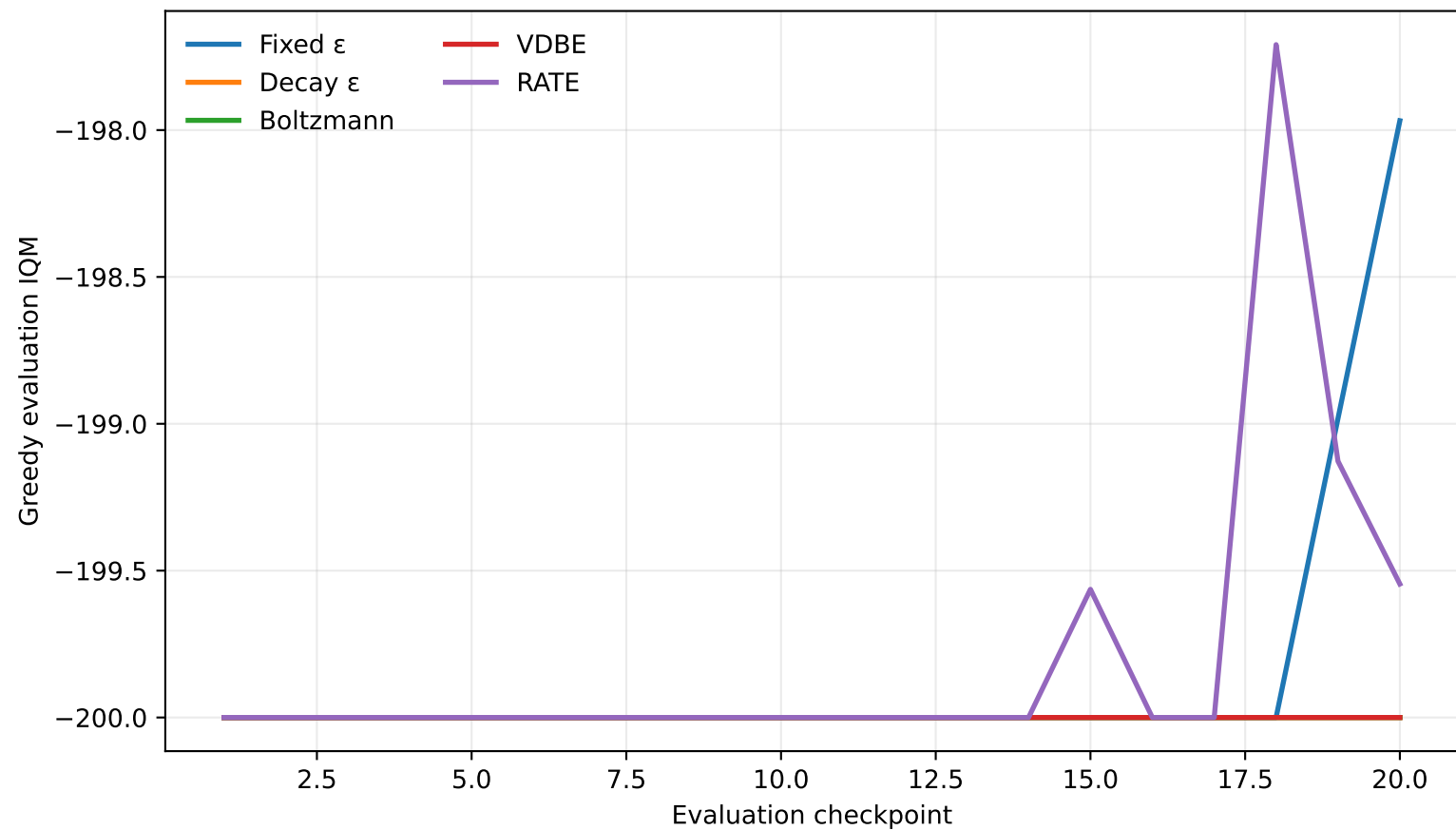
MountainCar — Double DQN
