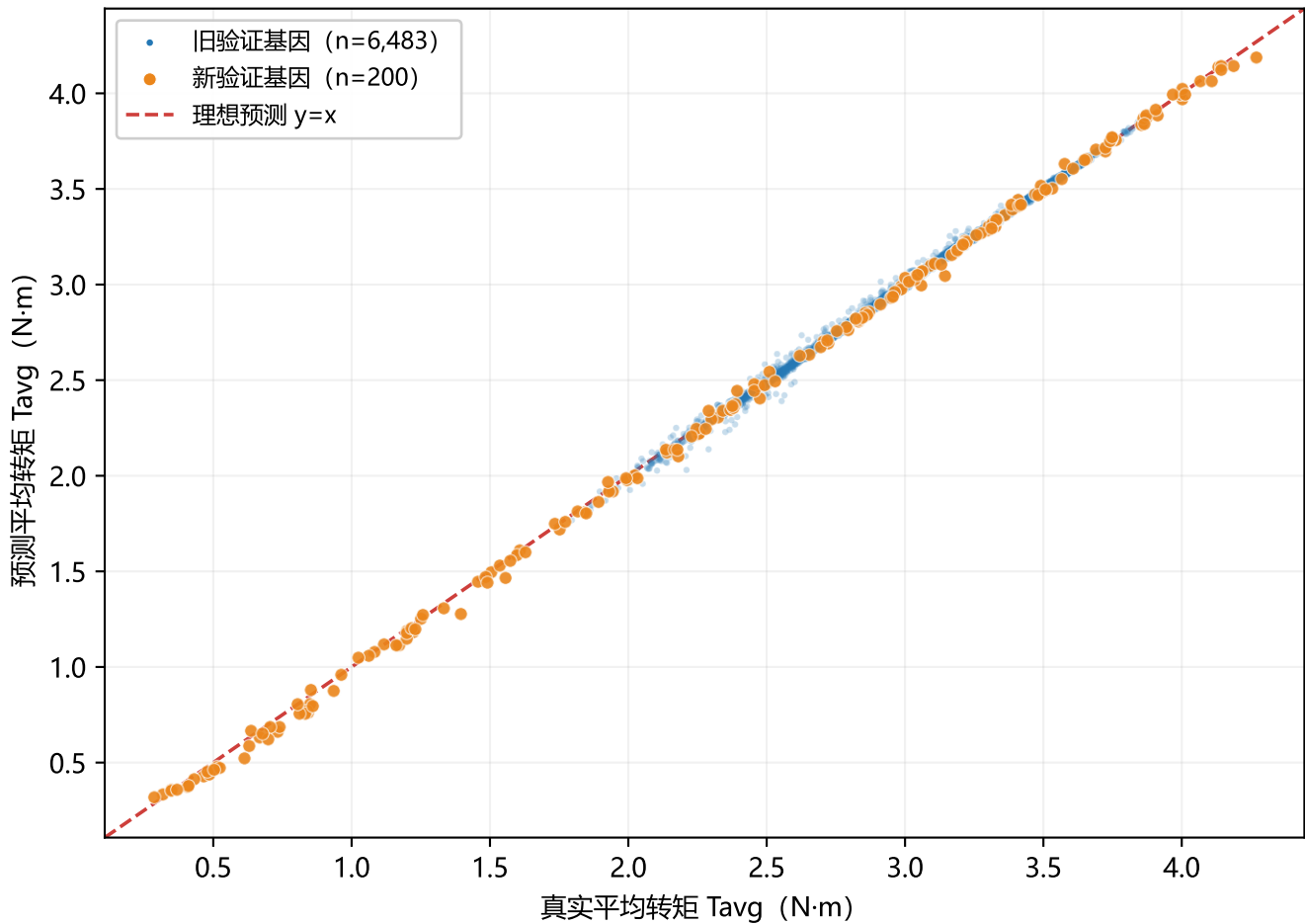
F-S 更新模型 · 新验证最优检查点（1500步）
