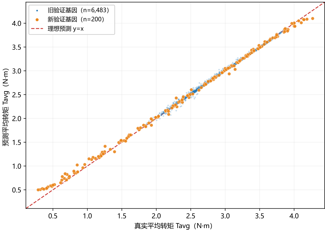
G-S 更新模型 · 新验证最优检查点（2000步）
