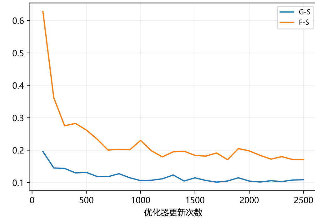
补样训练标准化 MSE (100步均值)
