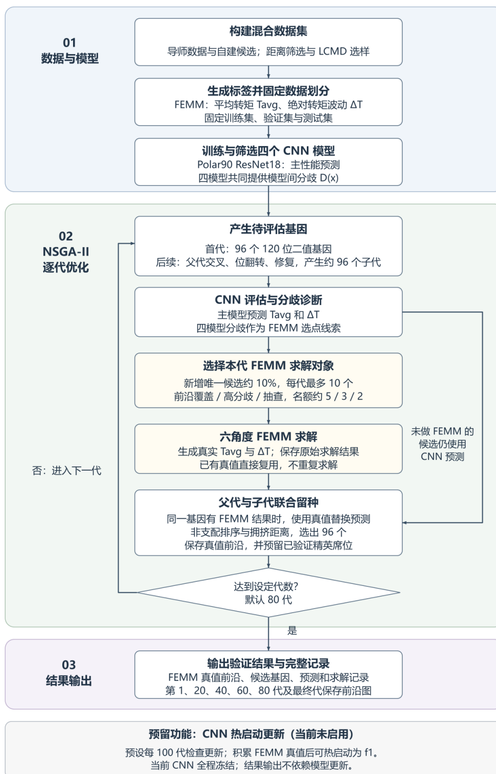
图 1-1 SPMSM 数据驱动多目标优化总体流程（中文版）
