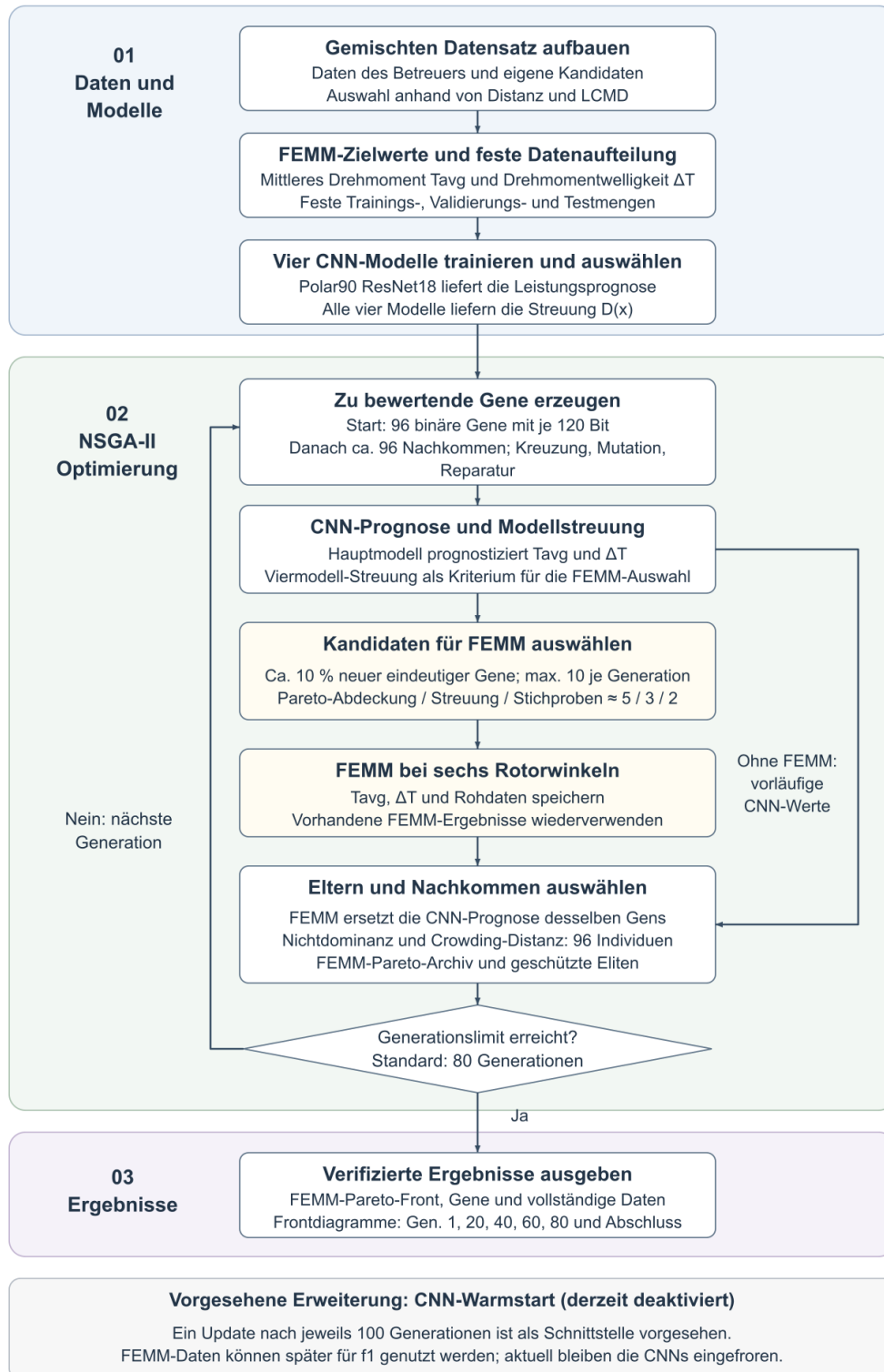
Abbildung 1-2 Gesamtprozess der datengetriebenen SPMSM-Optimierung
