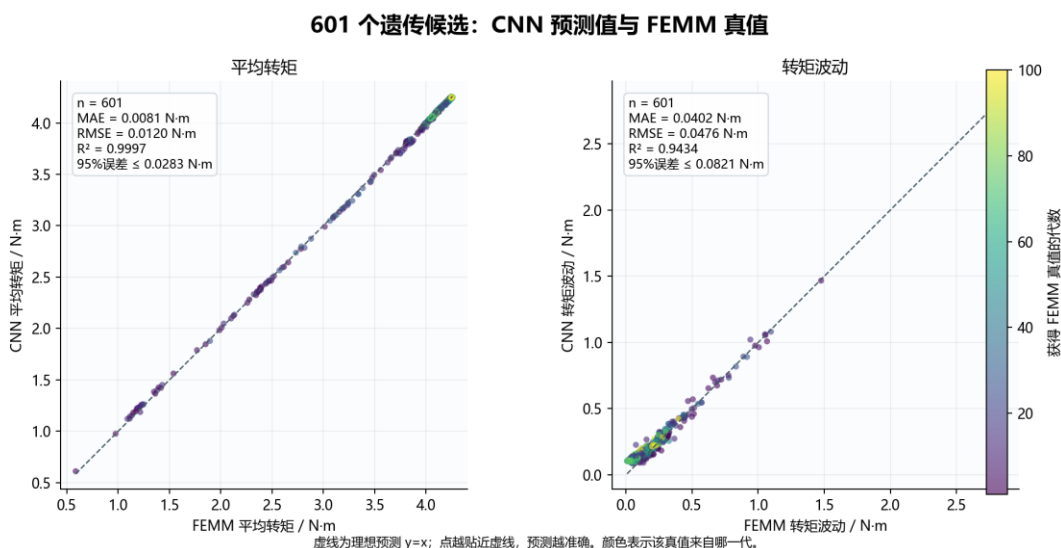
图 7-2 601 个遗传候选的 CNN 预测值与 FEMM 真值对比
