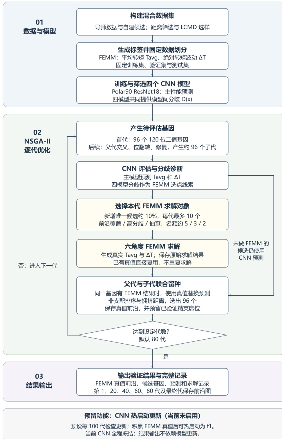
图 1-1 SPMSM 数据驱动多目标优化总体流程（中文版；图中 80 代为初始方案，本轮实际运行 100 代）
