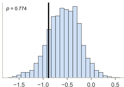
PyDescriptor (62571)
