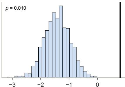
PaDEL (1444)
