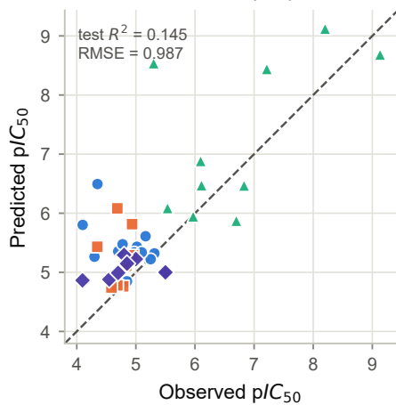
DFT+MD (381)
