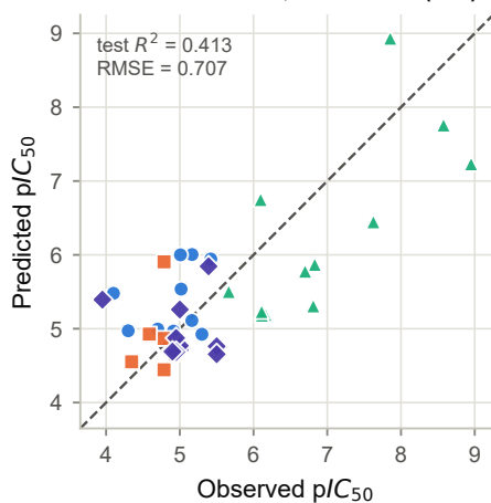
MD + PaDEL (1549)
