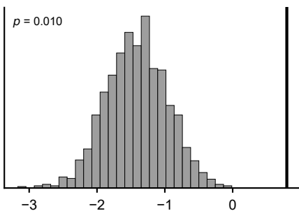
PaDEL (1444)
