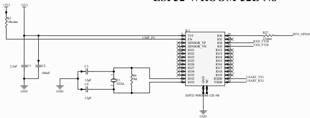
ESP32-WROOM-32E-N8
