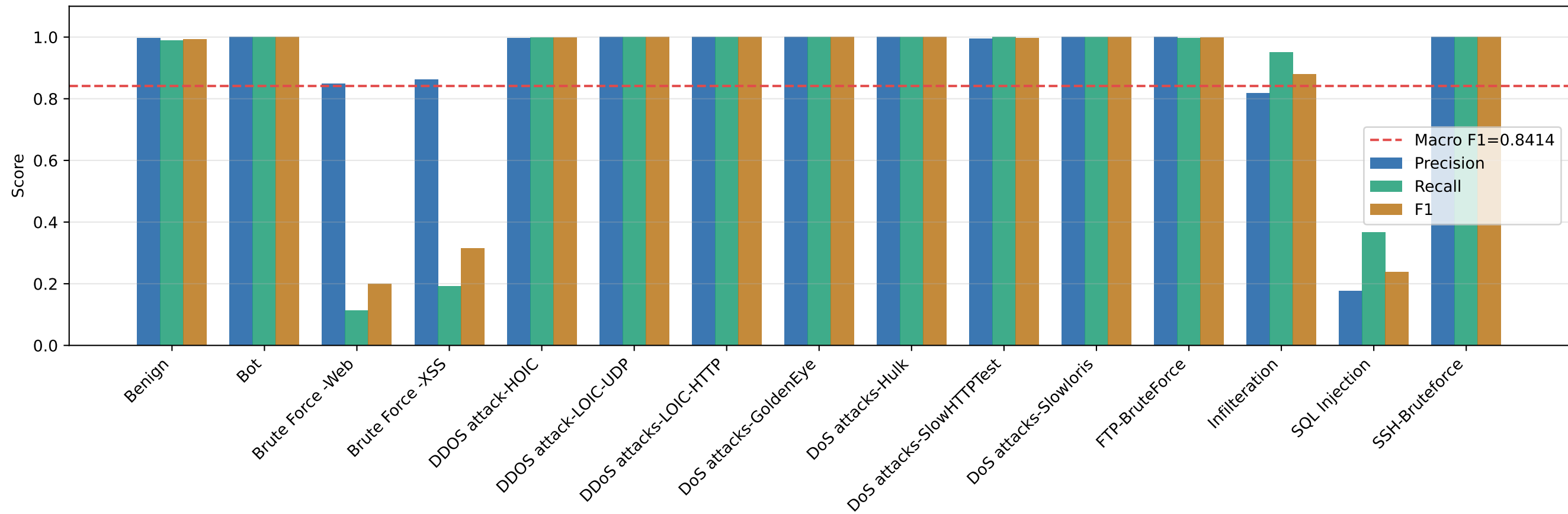
Per-class Precision / Recall / F1 — Test Set
