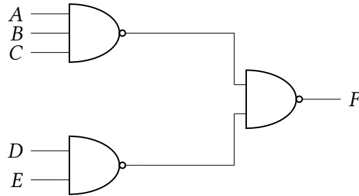
Şekil 2.20: Kaskad NAND kapılarıyla F = [(ABC)'(DE)']' = ABC + DE gerçeeklemesi.
