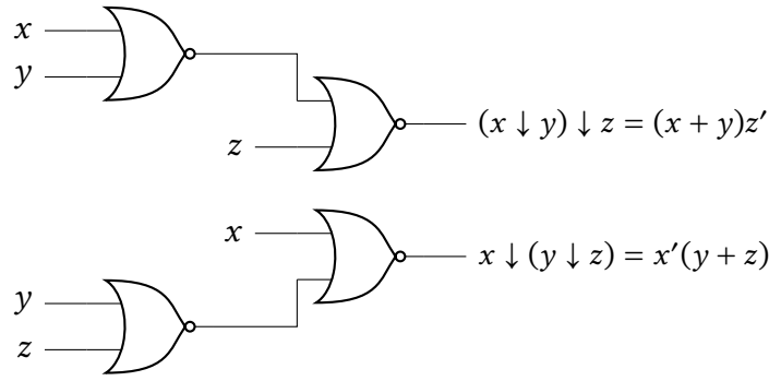
Şekil 2.18: NOR işleminin birleşmeli olmadığı gösterimi: (x \downarrow y) \downarrow z \neq x \downarrow (y \downarrow z) .
