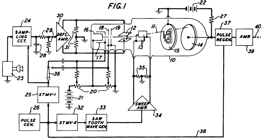
Şekil 1.7: Gray’in 2,632,058 numaralı patentinin ön sayfasından bir bölüm; yansıtılmış ikili kodu taşıyan plakayı (15) içeren PCM tüpü (10) görülüyor.
