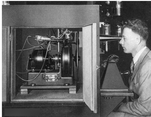
Şekil 1.6: Frank Gray, 1930'da geliştirdiği mekanik televizyon aygıtını incelerken.
