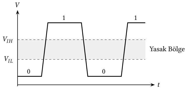
Şekil 1.3: Zamanla değişen bir dijital sinyal: yüksek/düşük seviyeler ve aradaki yasak bölge.
