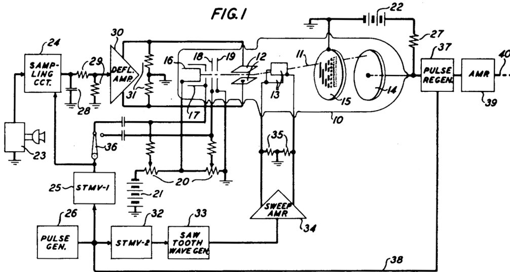
Şekil 1.8: Gray'ın 2,632,058 numaralı patentinin ön sayfasından bir bölüm; yansıtılmış ikili kodu taşıyan plakayı (15) içeren PCM tüpü (10) görülüyor.
