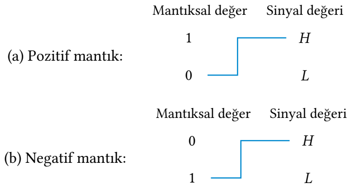
Şekil 2.30: Mantıksal değerin sinyal değerine ataması.
