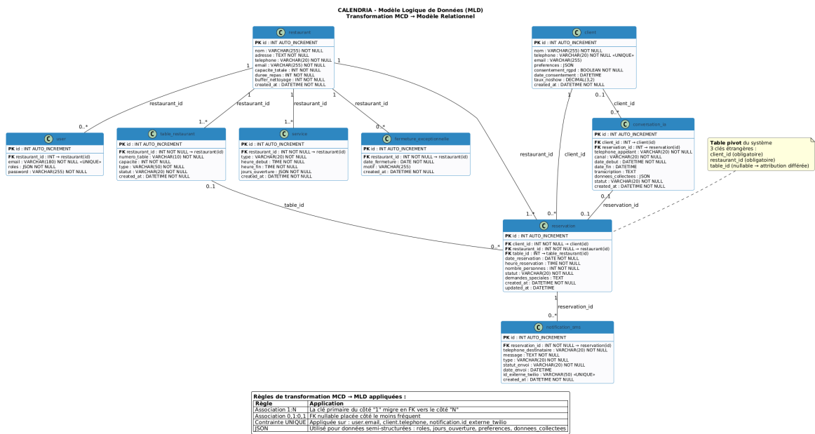
Figure 6.2 - Modèle Logique de Données (MLD)
