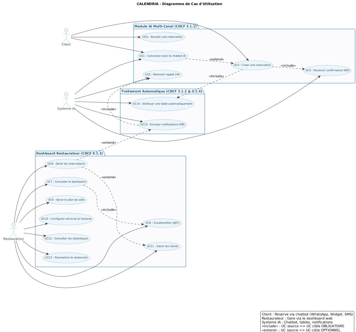
Figure 7.1 - Diagramme des Cas d'Utilisation
