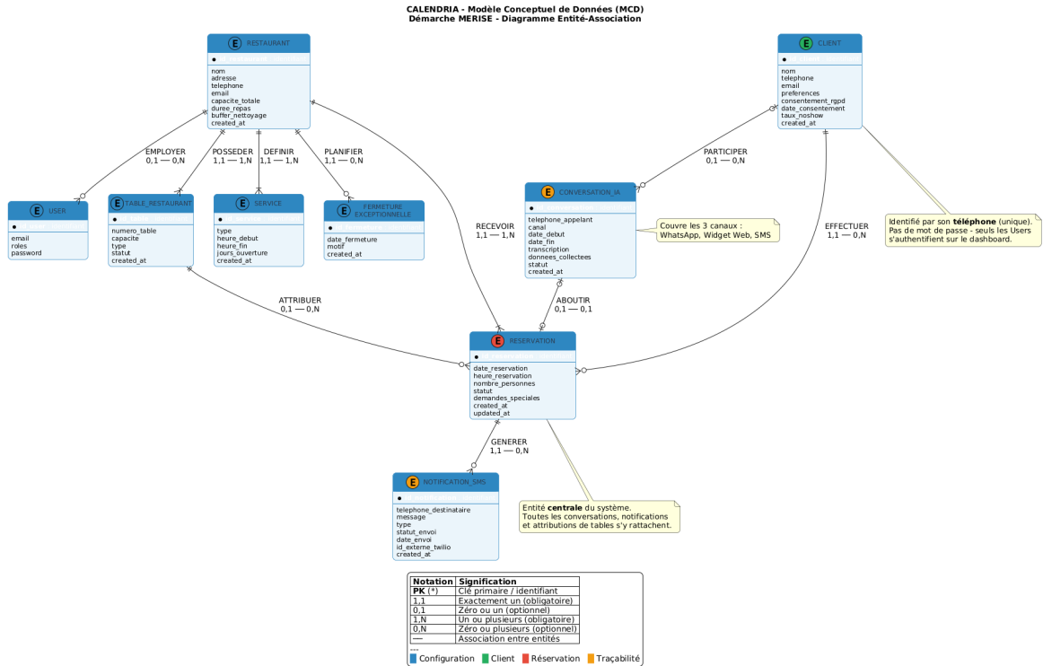
Figure 6.1 - Modèle Conceptuel de Données (MCD)
