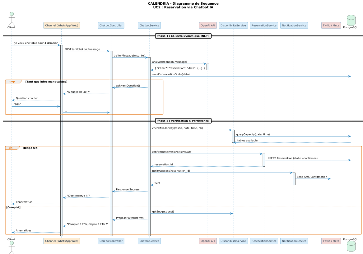
Figure 7.2 - Séquence Réservation via Chatbot IA
