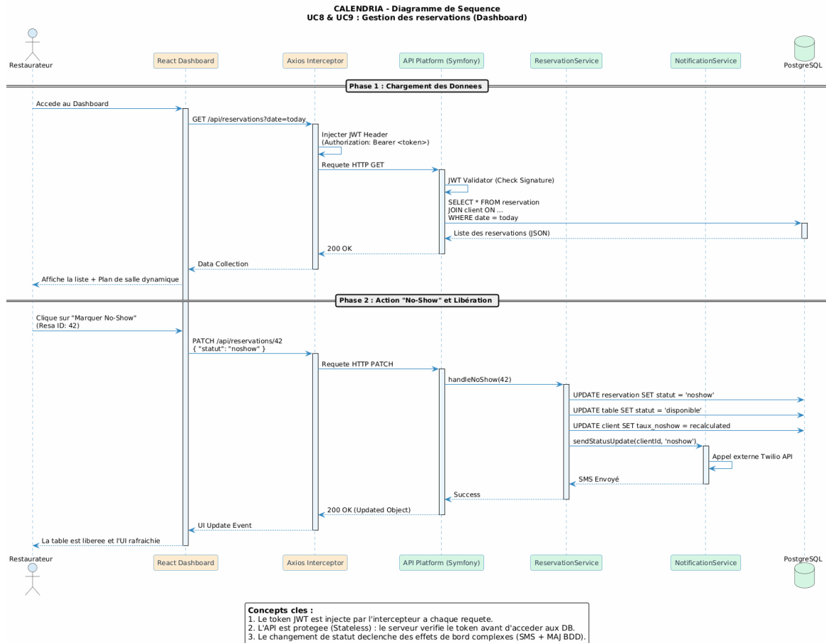
Figure 7.4 - Séquence Gestion Réservation
