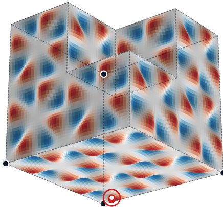
B: k = (0, 2, 1) , e = (1, 0, 0)
