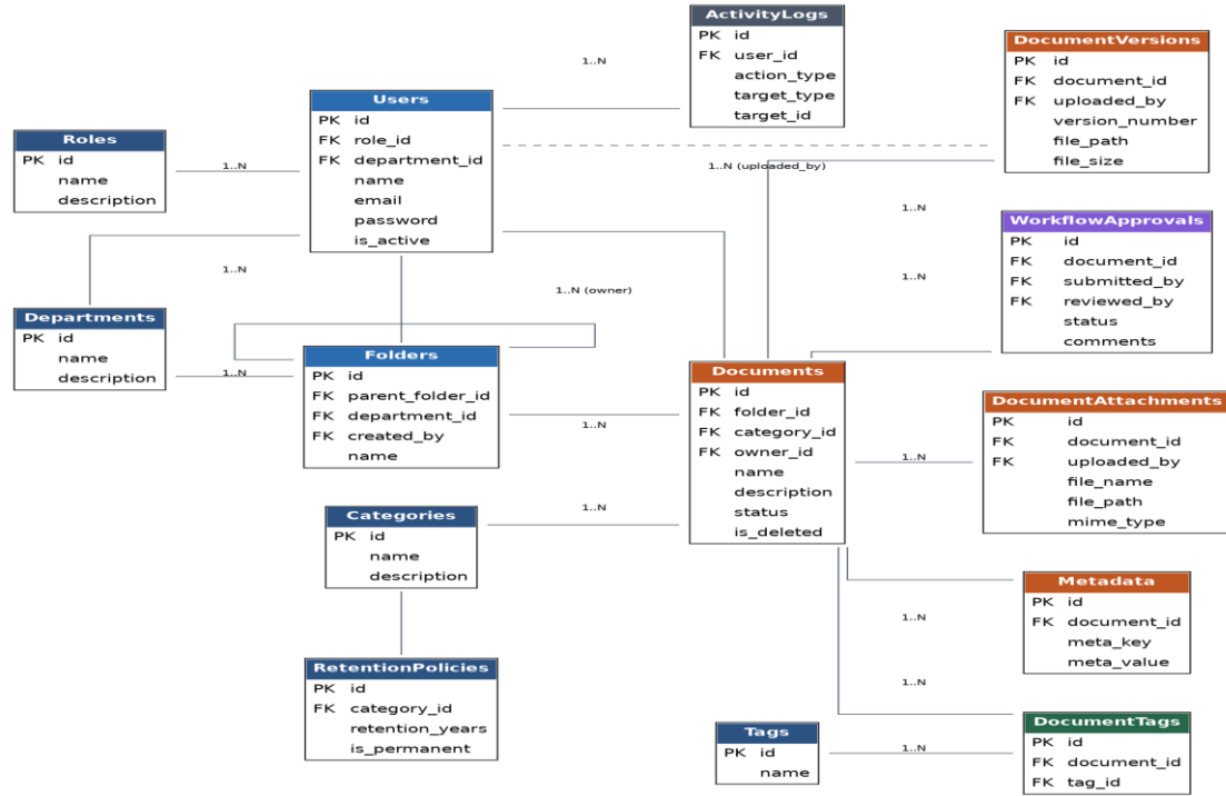
لنظام إدارة المستندات (ERD) الشكل 1: مخطط علاقات الكيانات
