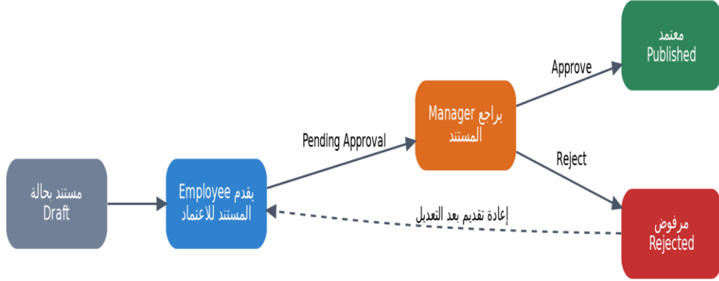
الشكل 3: دورة حياة سير عمل اعتماد المستند
