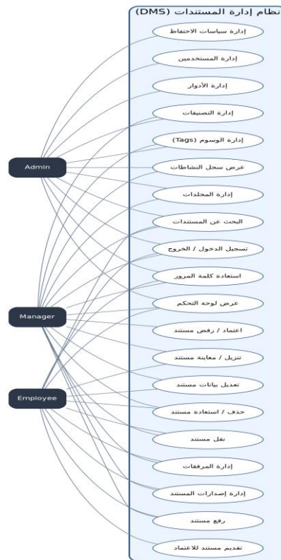
الشكل 2: مخطط حالات الاستخدام لنظام إدارة المستندات
