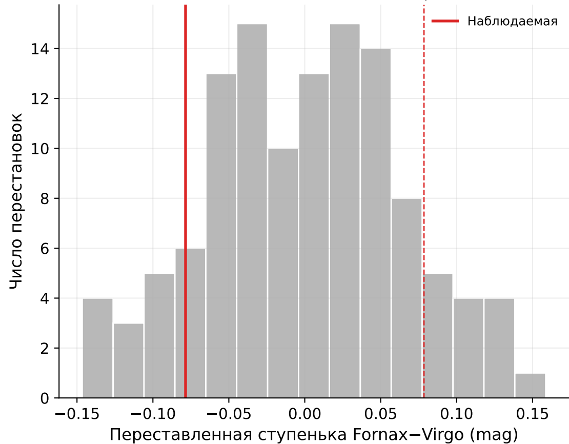
Точный тест меток скоплений: p=0.233
