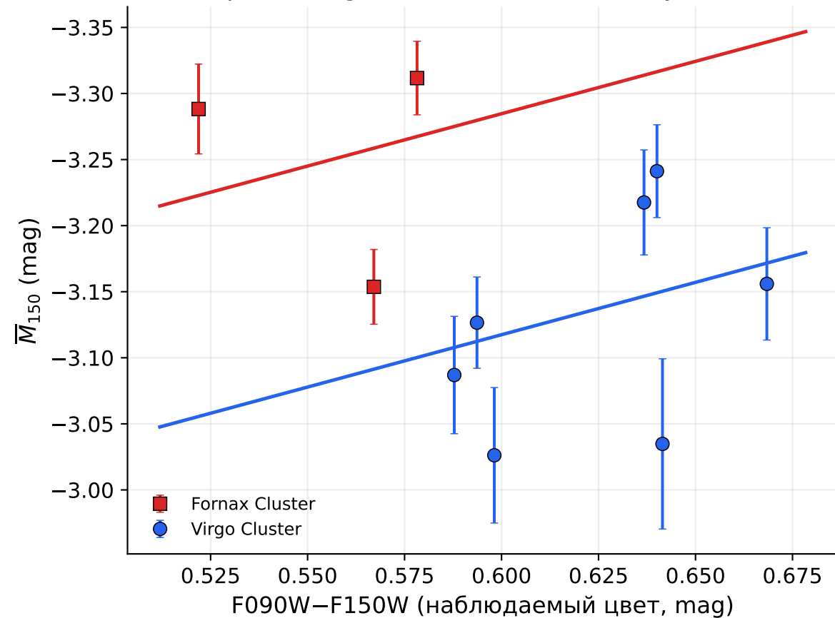
Строгие Virgo и Fornax: наклон + ступенька
