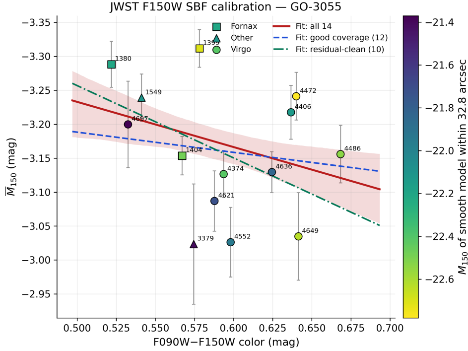
Рис. 1: Прямая калибровка JWST F150W SBF для GO-3055. Форма маркера показывает окружение, цвет — апертурную светимость гладкой модели. Вертикальная ось перевернута: более яркие SBF расположены выше.
