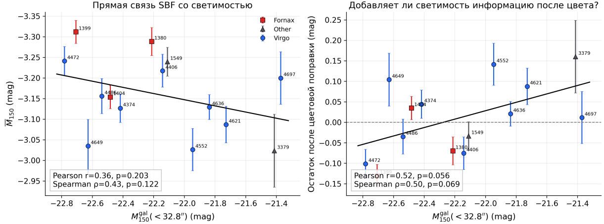
Рис. 5: Абсолютная F150W SBF-величина и остаток после цветовой поправки в зависимости от абсолютной F150W-величины гладкой модели галактики внутри 32.8 угл. сек. Правая панель проверяет, добавляет ли светимость информацию после учёта цвета.
