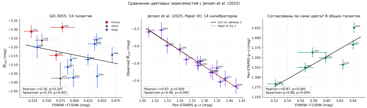
Рис. 2: Слева и в центре: наблюдаемые зависимости абсолютной SBF-величины от цвета для настоящей работы и Paper III. Справа: прямое сравнение F090W–F150W и g - z для восьми общих галактик. Наклоны первых двух панелей нельзя сравнивать буквально из-за разных SBF-фильтров и цветовых индексов.
