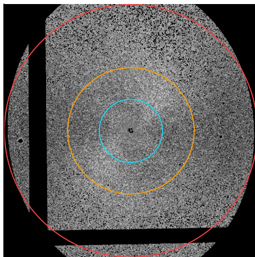
NGC 4621
