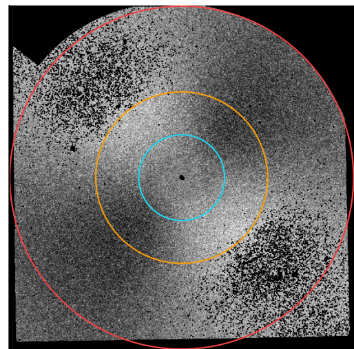
NGC 4636
