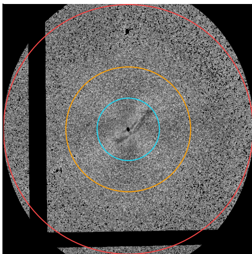
NGC 4552
