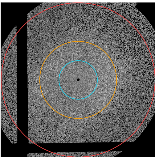
NGC 4486
