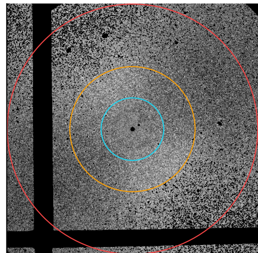
NGC 4636
