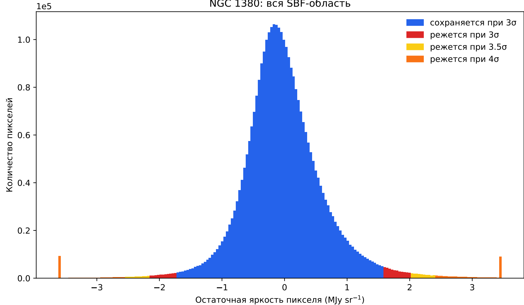
NGC 1380: вся SBF-область
