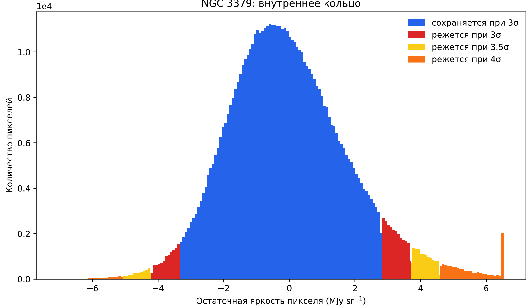
NGC 3379: внутреннее кольцо
