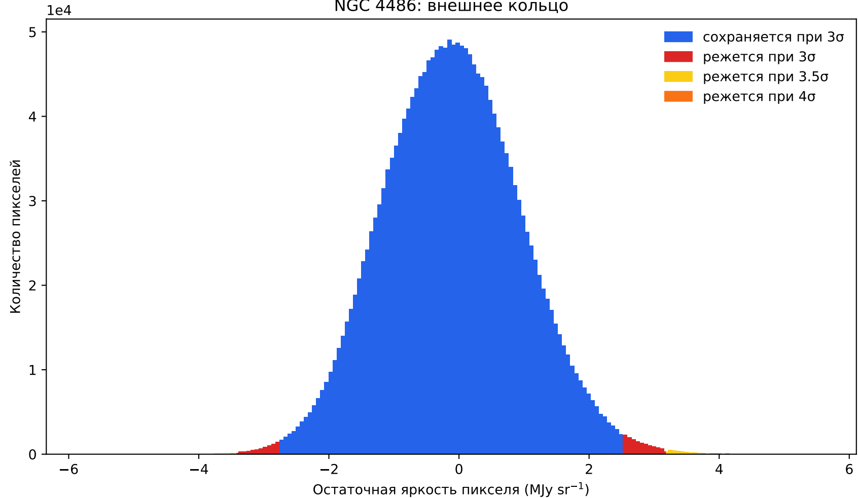
NGC 4486: внешнее кольцо
