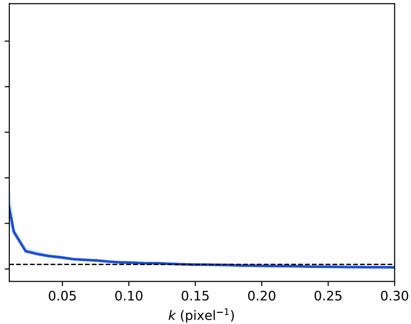
NGC 1380
