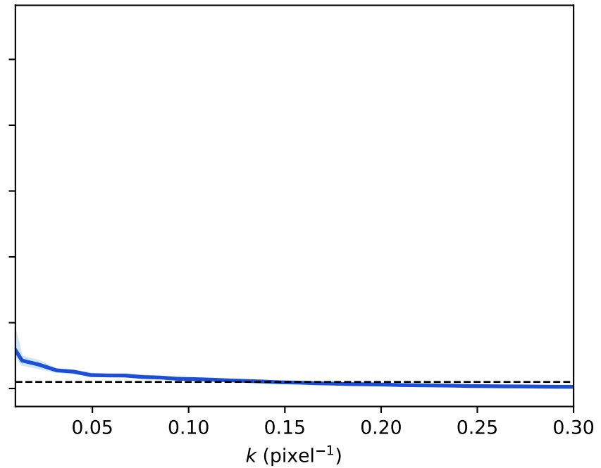
NGC 4486
