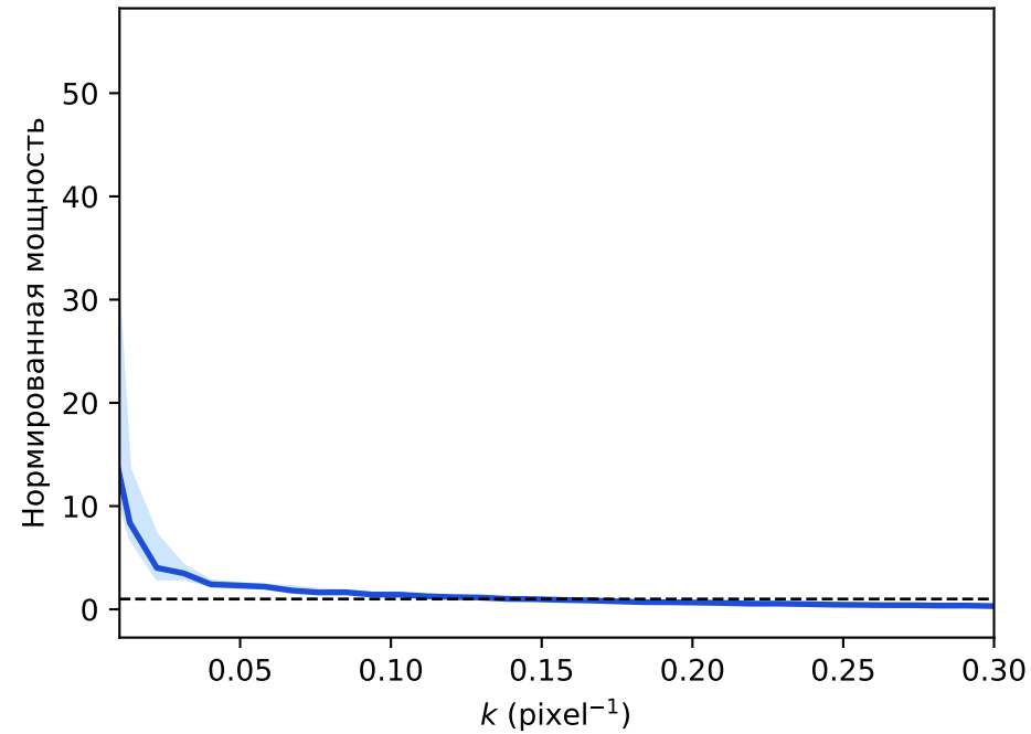
NGC 3379
