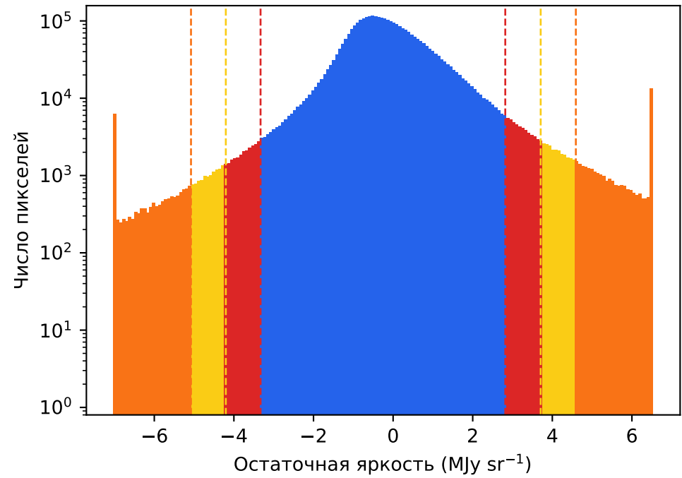
NGC 3379
