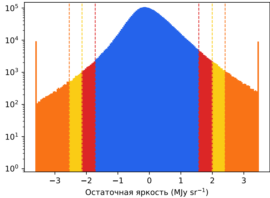
NGC 1380
