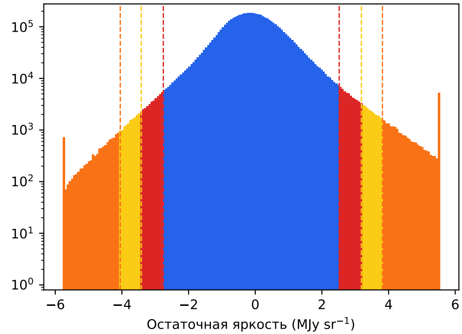
NGC 4486
