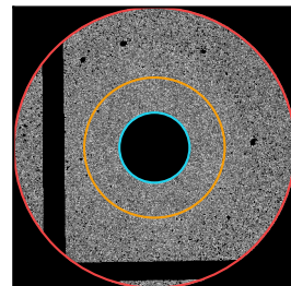
NGC 4636
