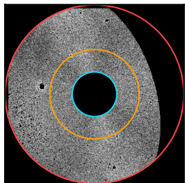
NGC 3379
