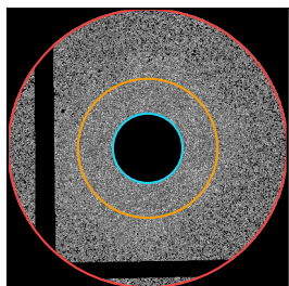
NGC 4486
