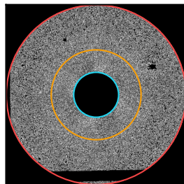
NGC 4406
