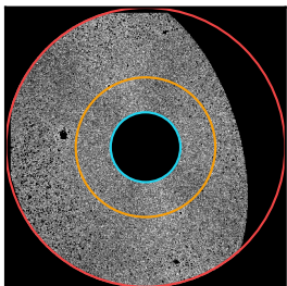
NGC 3379
