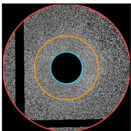
NGC 4486
