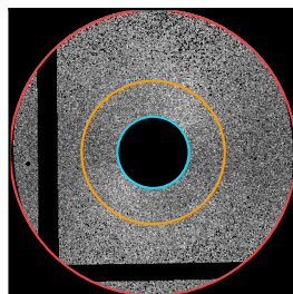
NGC 4621
