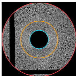
NGC 4697
