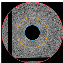
NGC 4552
