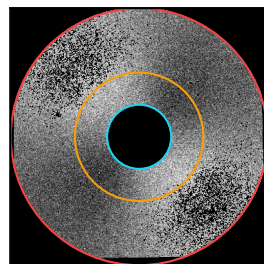
NGC 4636
