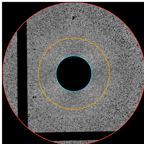
NGC 4552
