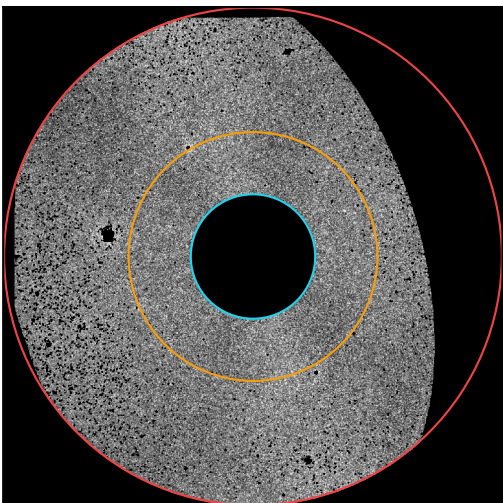
NGC 3379
