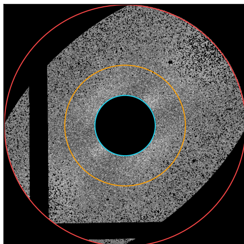
NGC 4697
