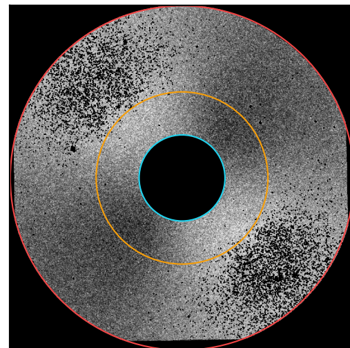
NGC 4636
