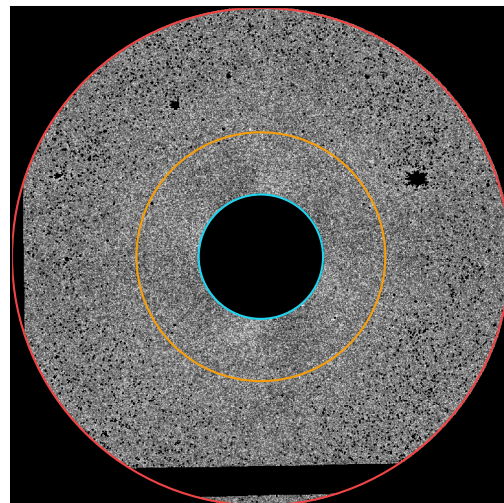
NGC 4406
