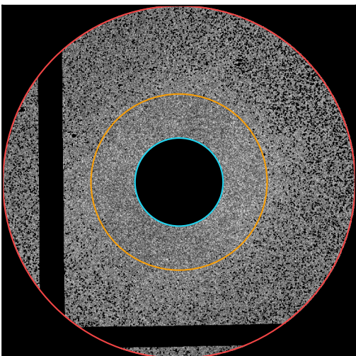
NGC 4486
