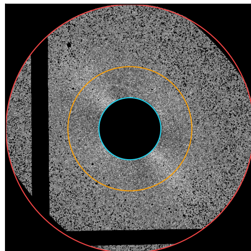
NGC 4621
