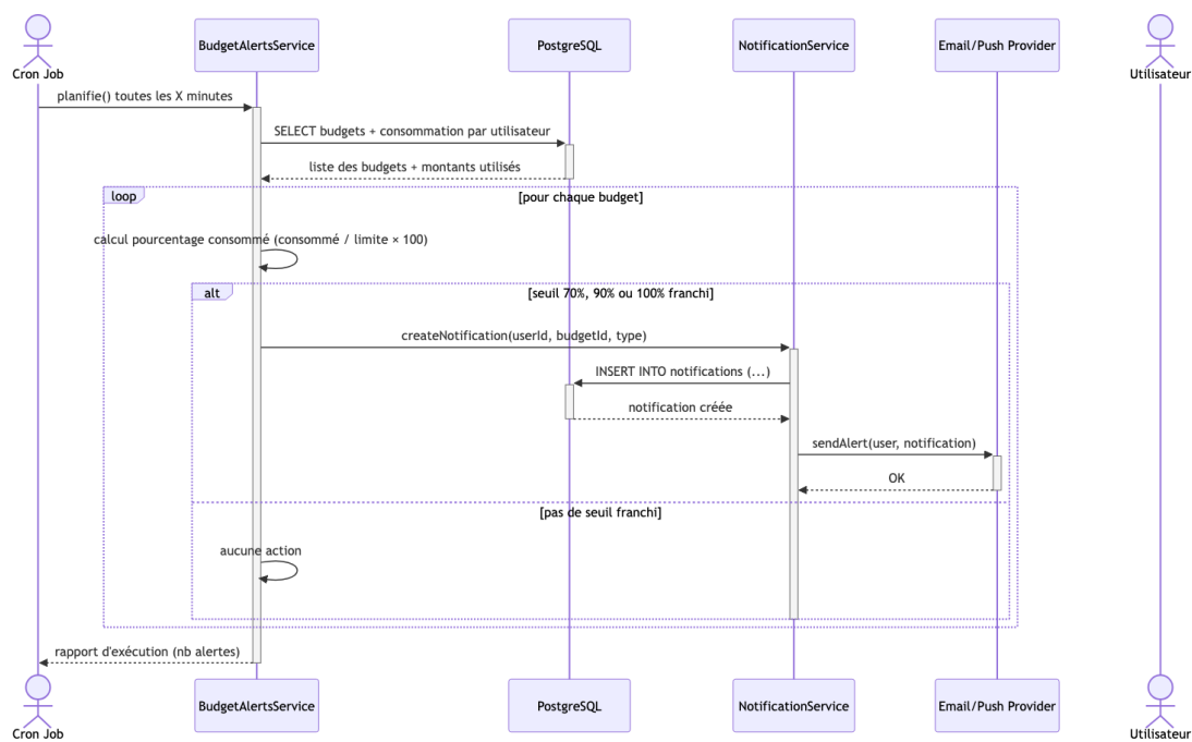
Figure A.17 – Diagramme de séquence — Flux automatique de déclenchement d’alertes
