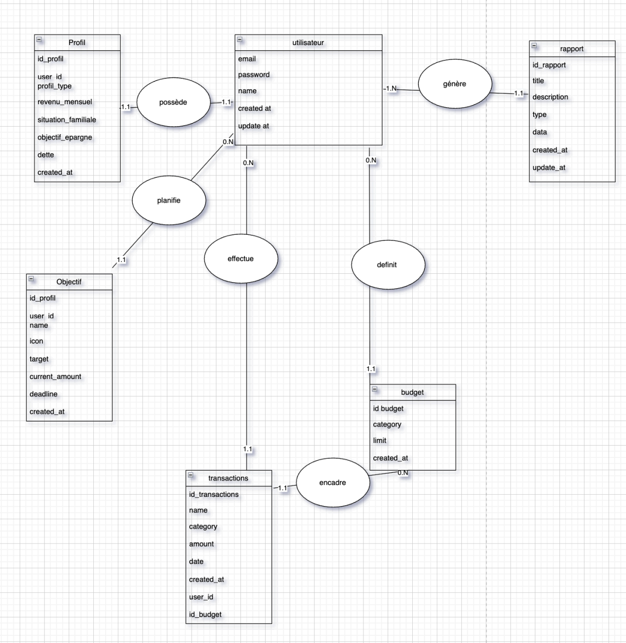
Figure A.20 – Modèle Conceptuel de Données (MCD) — entités et relations
