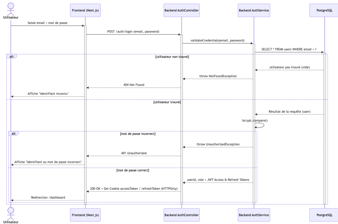
Figure A.15 – Diagramme de séquence — Flux de connexion utilisateur (Login)
