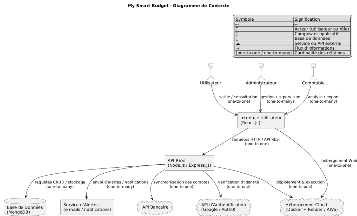
Figure 1.1 Diagramme de contexte – My Smart Budget
