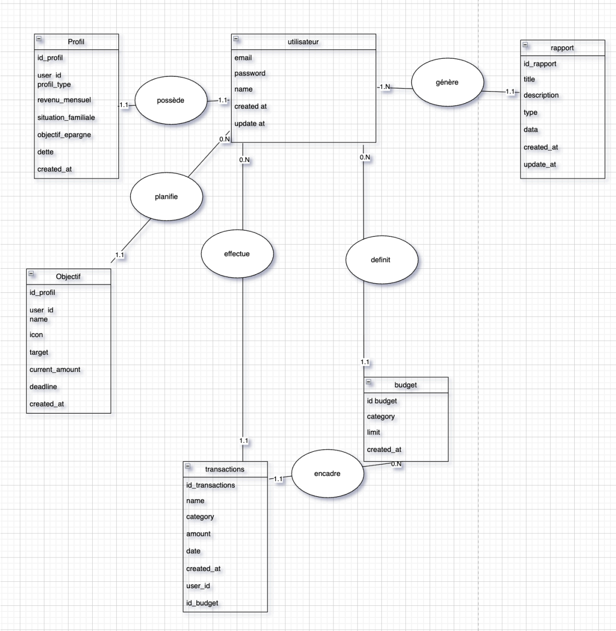
Figure A.19 Modèle Conceptuel de Données (MCD) – entités et relations
