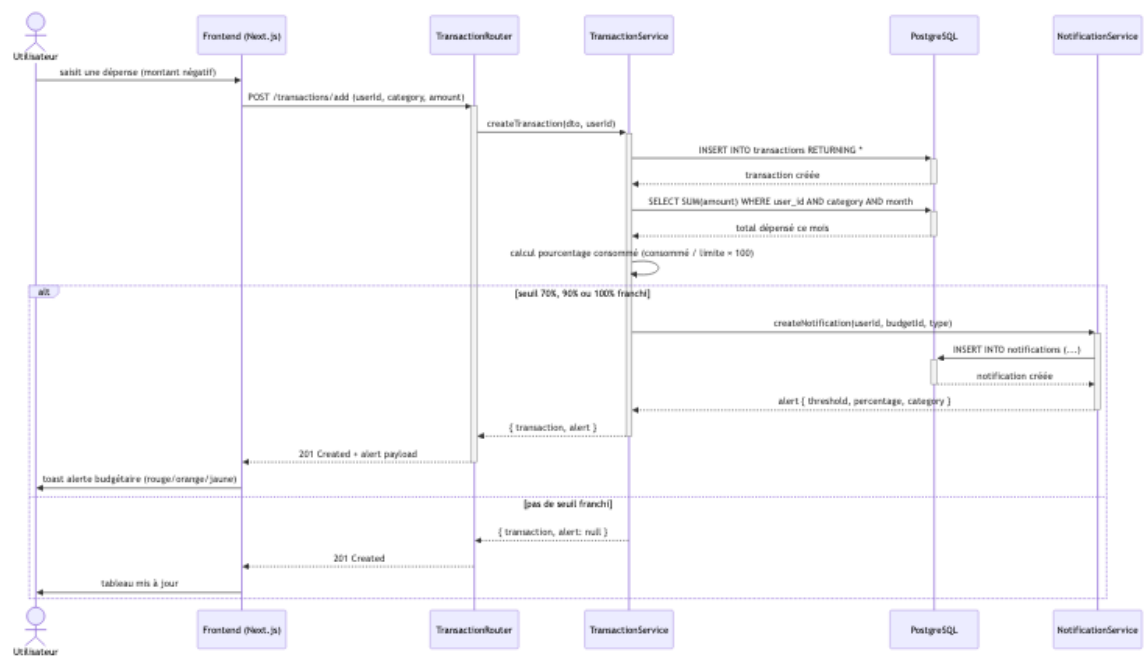
Figure A.16 Diagramme de séquence – Flux automatique de déclenchement d’alertes
