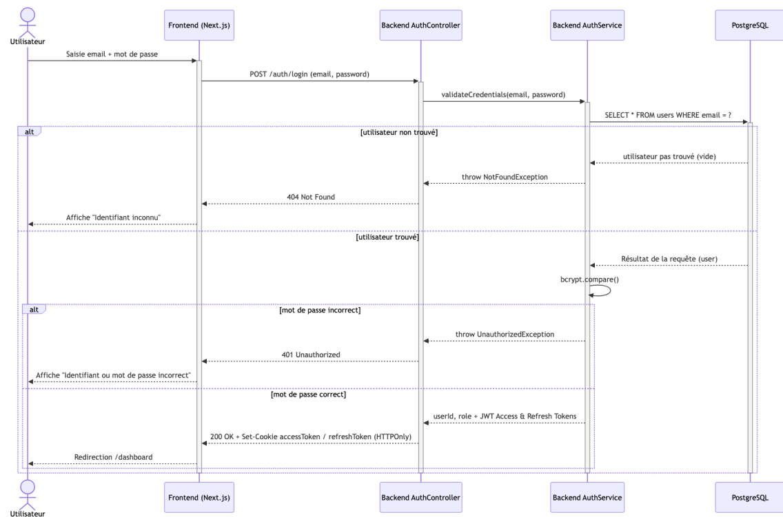
Figure A.14 Diagramme de séquence – Flux de connexion utilisateur (Login)
