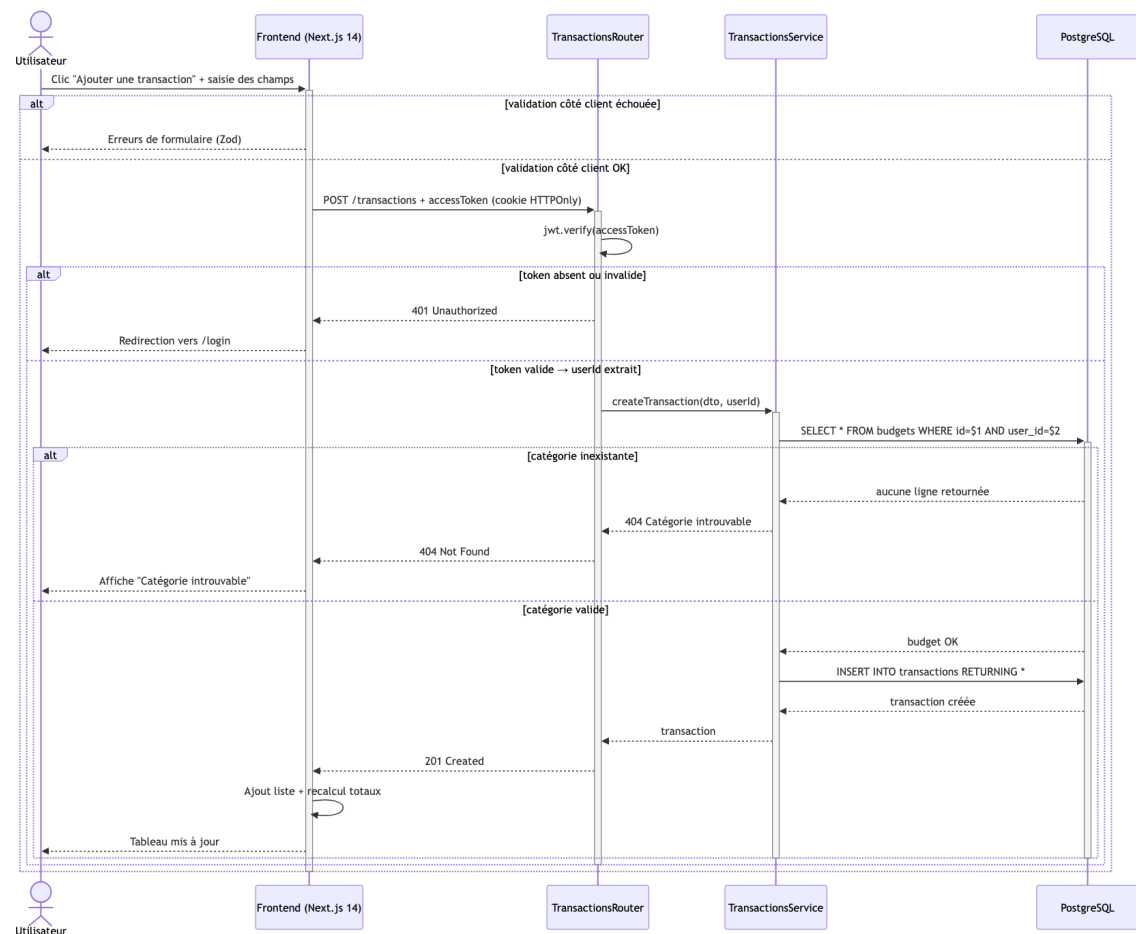
Figure A.15 Diagramme de séquence – Flux de création d'une transaction
