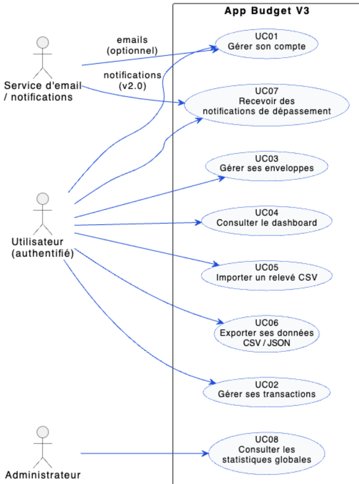
Figure A.13 – Diagramme de cas d'usage global — App Budget V3
