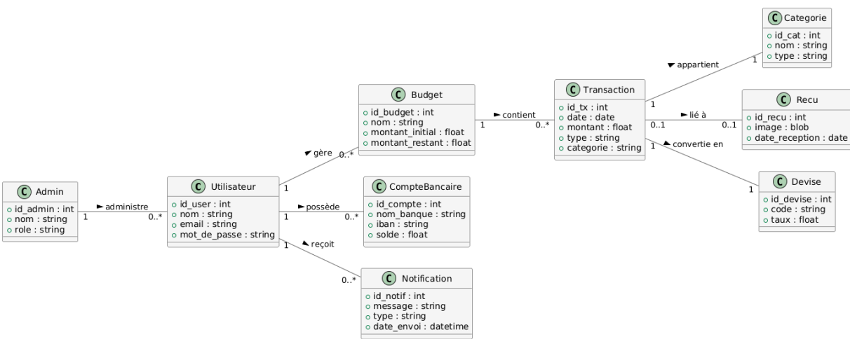
Figure A.2 – Diagramme de classes UML de l'application My Smart Budget
