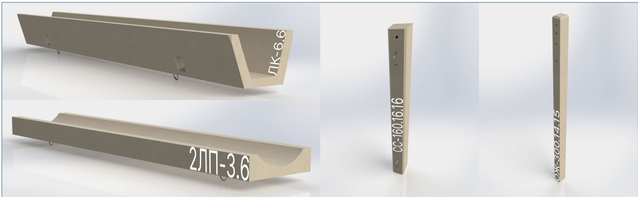
Лотки кюветные, прикромочные, сигнальный столбик и ж/б опоры дорожных знаков
