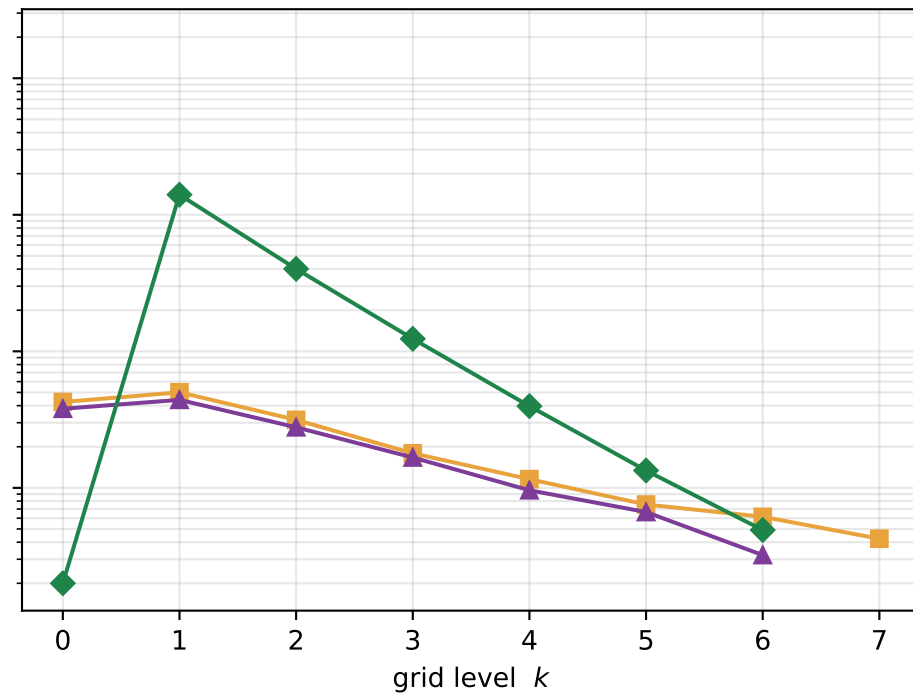
precision correction (odd l = 2k + 1 )
