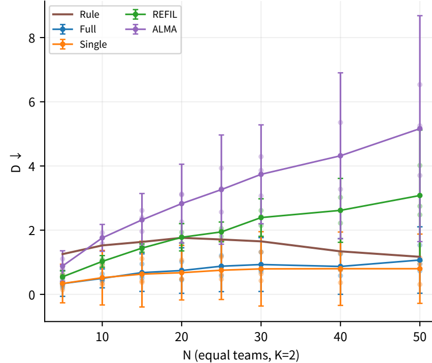
e. SMACv2 team-size transfer
