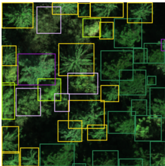
BBox
