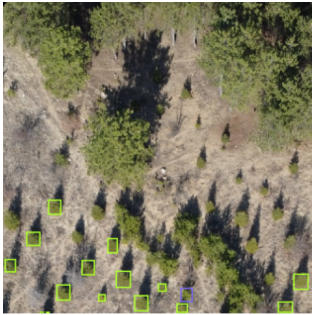
BBox
