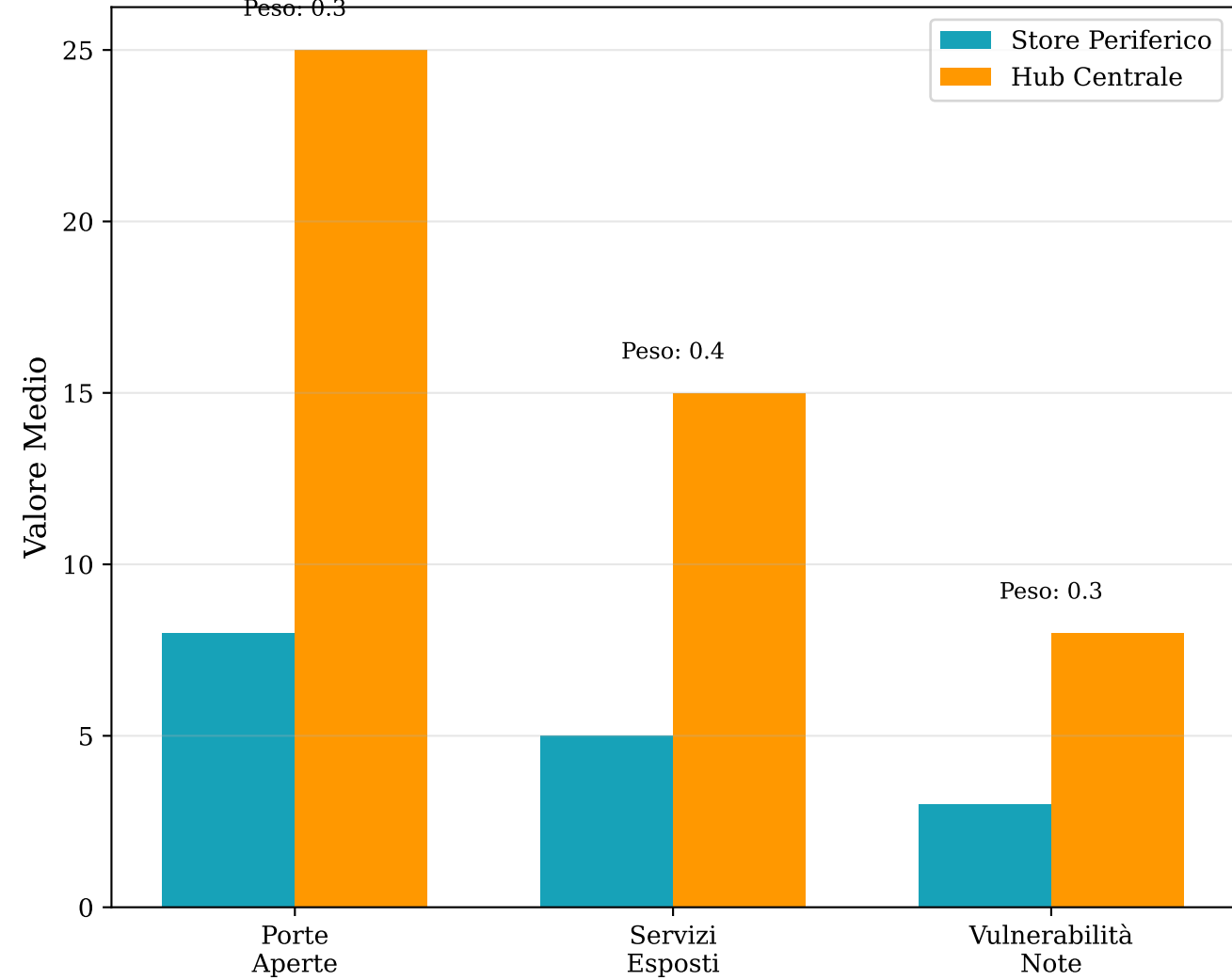
Componenti ASSA per Tipo di Nodo
